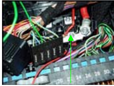
Anschluss Dauerstrom
