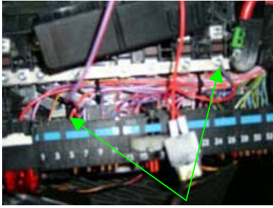
Anschluss Dauerstrom, Modul und Steckdose
