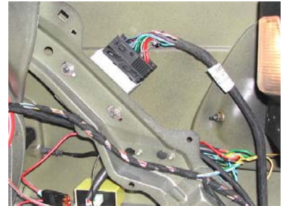
Einbau Modul
